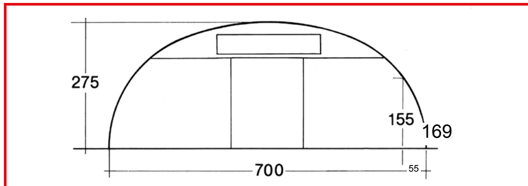
Filclair - Gewächshaus mit Konfektioniertem Schattiergewebe
