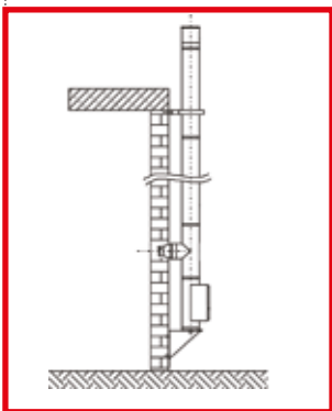
Doppelwandiger Schornstein für Außenmontage
