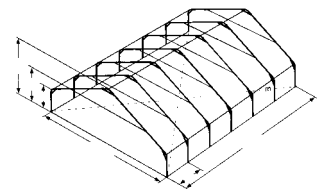
12 m-Haus, Stehwandhöhe 2,60 m, Rechteckbinder 120 x 60 x 6 mm, feuerverzinkt
